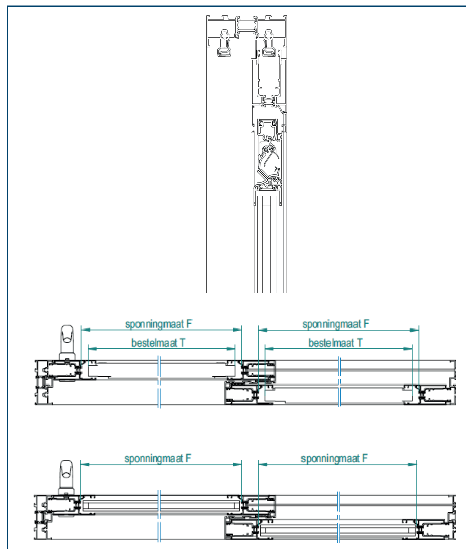
SlideStream 10 in een aluminium schuifpui
