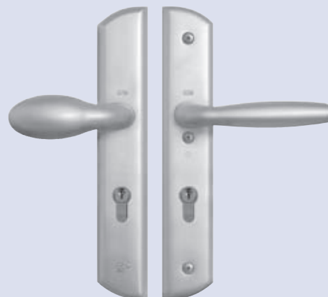
Serie 2815-GD, PC 92-uitvoering voor Ergo-Motion
