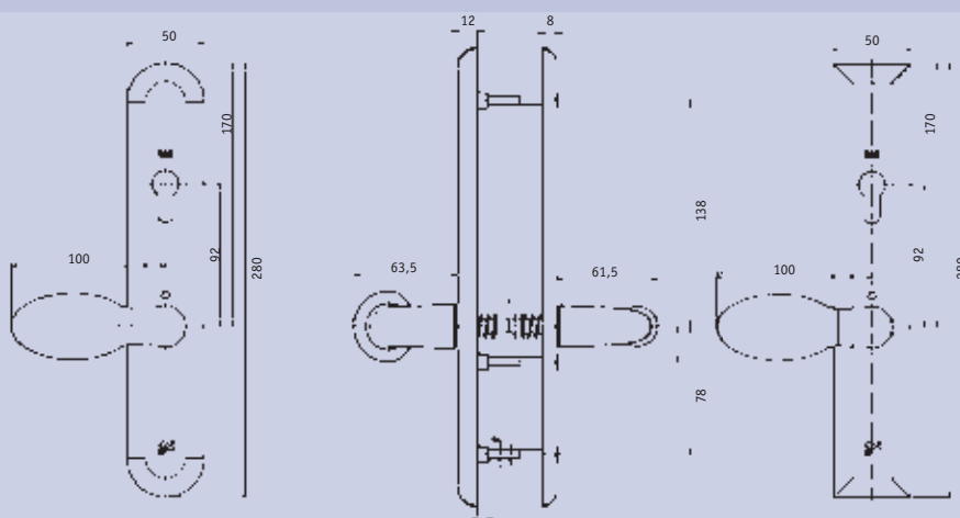
Serie 2831 (afgerond) en Serie 2851 (rechthoekig)
