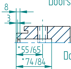
Doorsnede S-S
