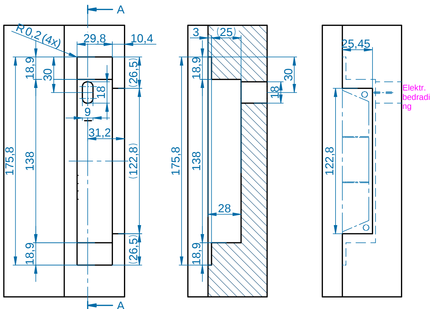
Doorsnede A-A
